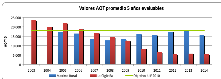
Gráfico 18.- Valor AOT40 de O 3 promedio de 5 años. Protección de los ecosistemas.
