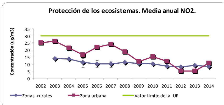
Gráfico 7.- Media anual \text{NO}_2 - Protección de los ecosistemas.
