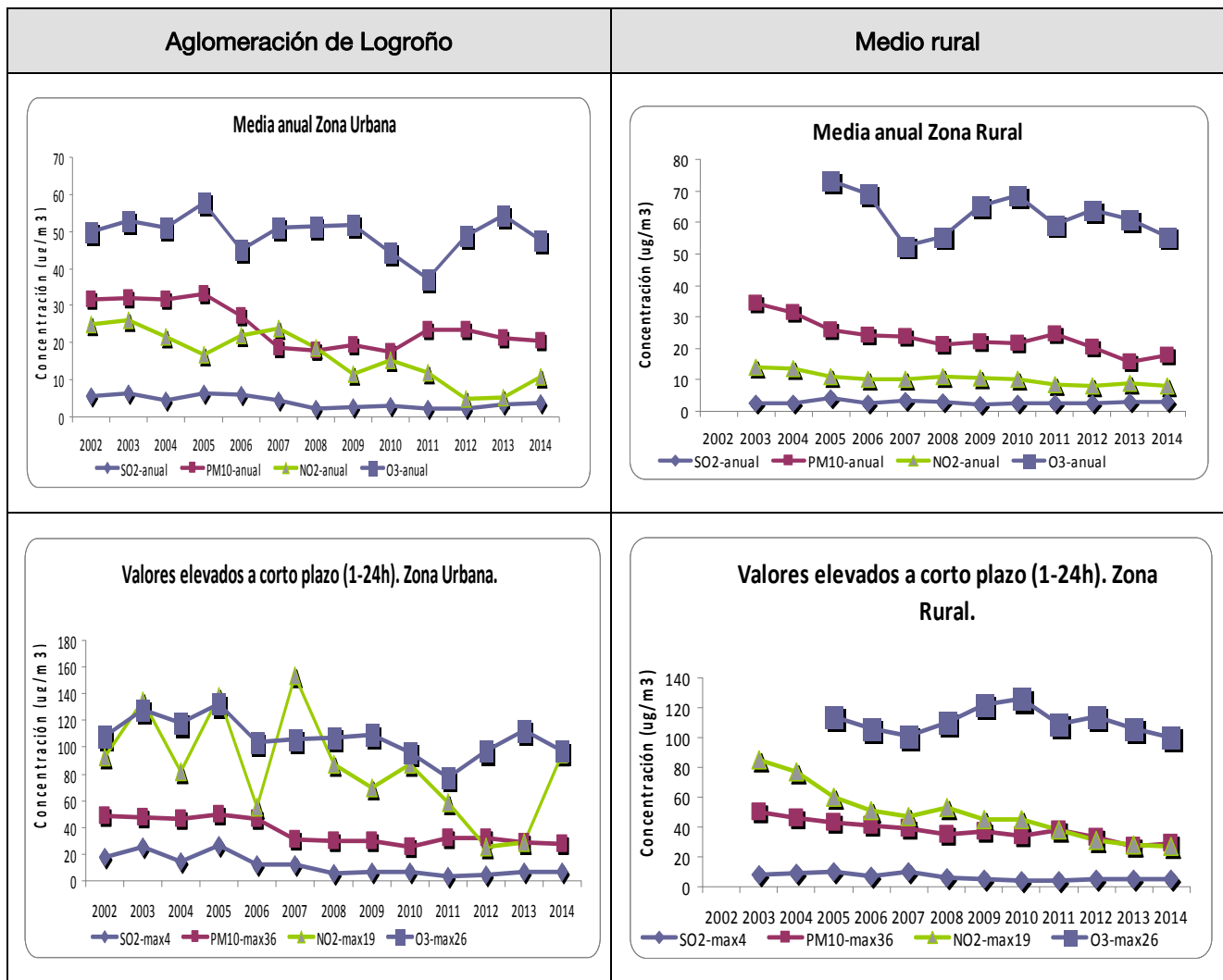
Gráfico 4.- Gráficas de tendencias de las concentraciones de contaminantes atmosféricos en zonas urbanas y rurales.
