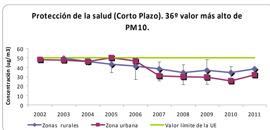
Gráfico 10.- 36º valor más alto PM 10 en todas las estaciones.
