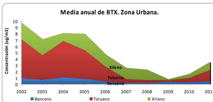
Gráfico 14.- Media anual BTX en Logroño.
