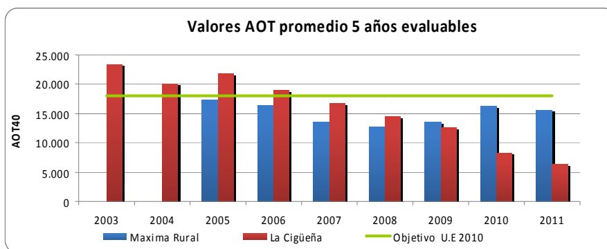
Gráfico 18.- Valor AOT40 de \text{O}_3 promedio de 5 años. Protección de los ecosistemas.
