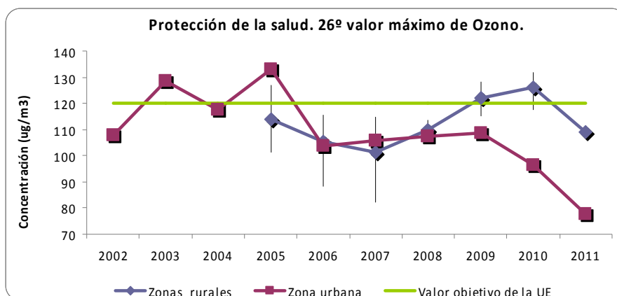
Gráfico 17.- 26º valor máximo de O 3 .
