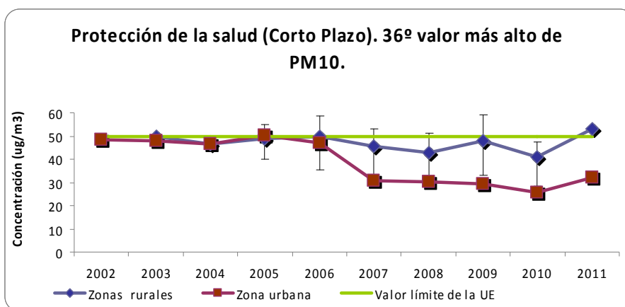
Gráfico 11.- 36º valor más alto PM 10 en todas las estaciones tomando los valores más desfavorables de las estaciones.
