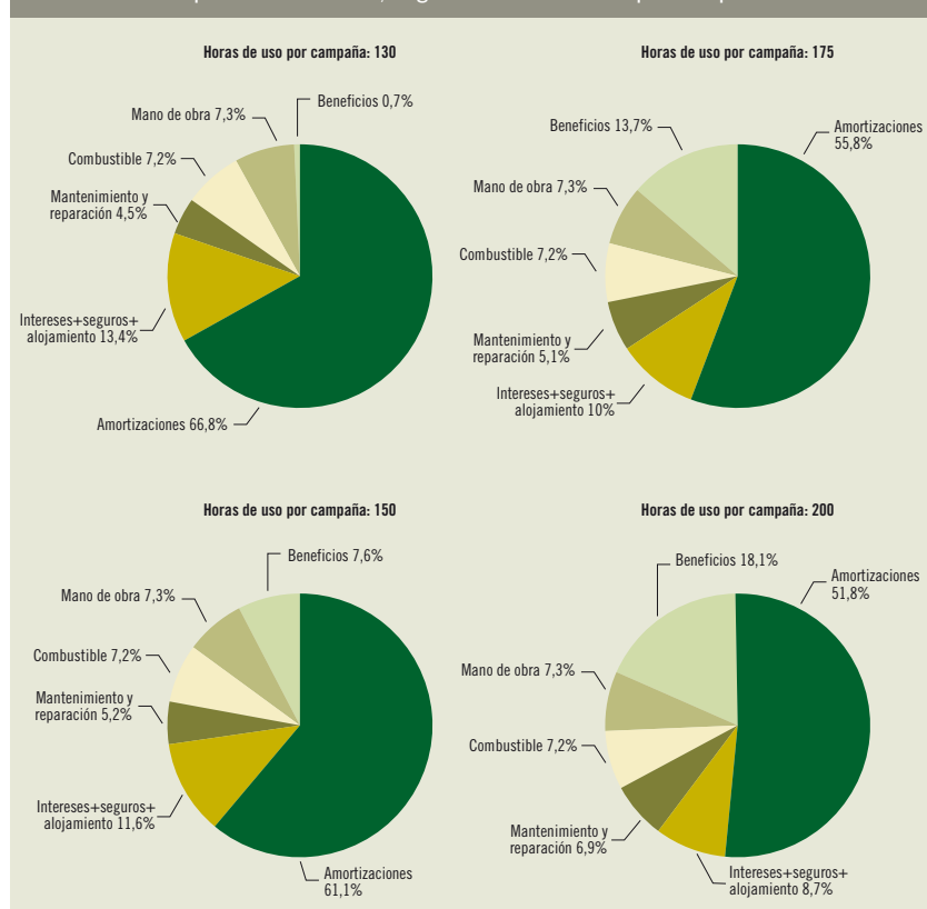
Gráfico 1. Distribución de los ingresos de una vendimiadora automotriz en una empresa de servicios, según las horas de uso por campaña
